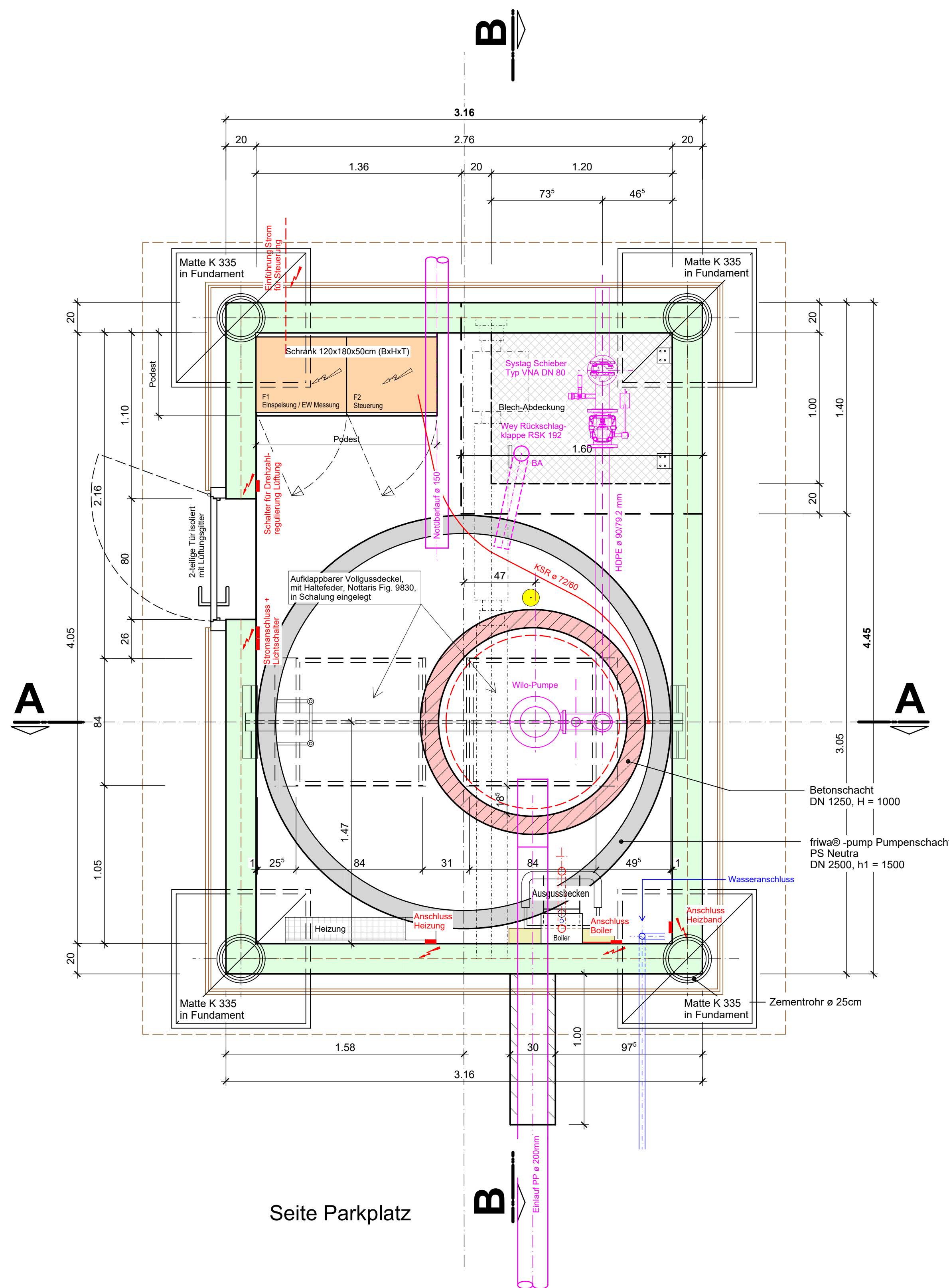
Grundriss 1:20
