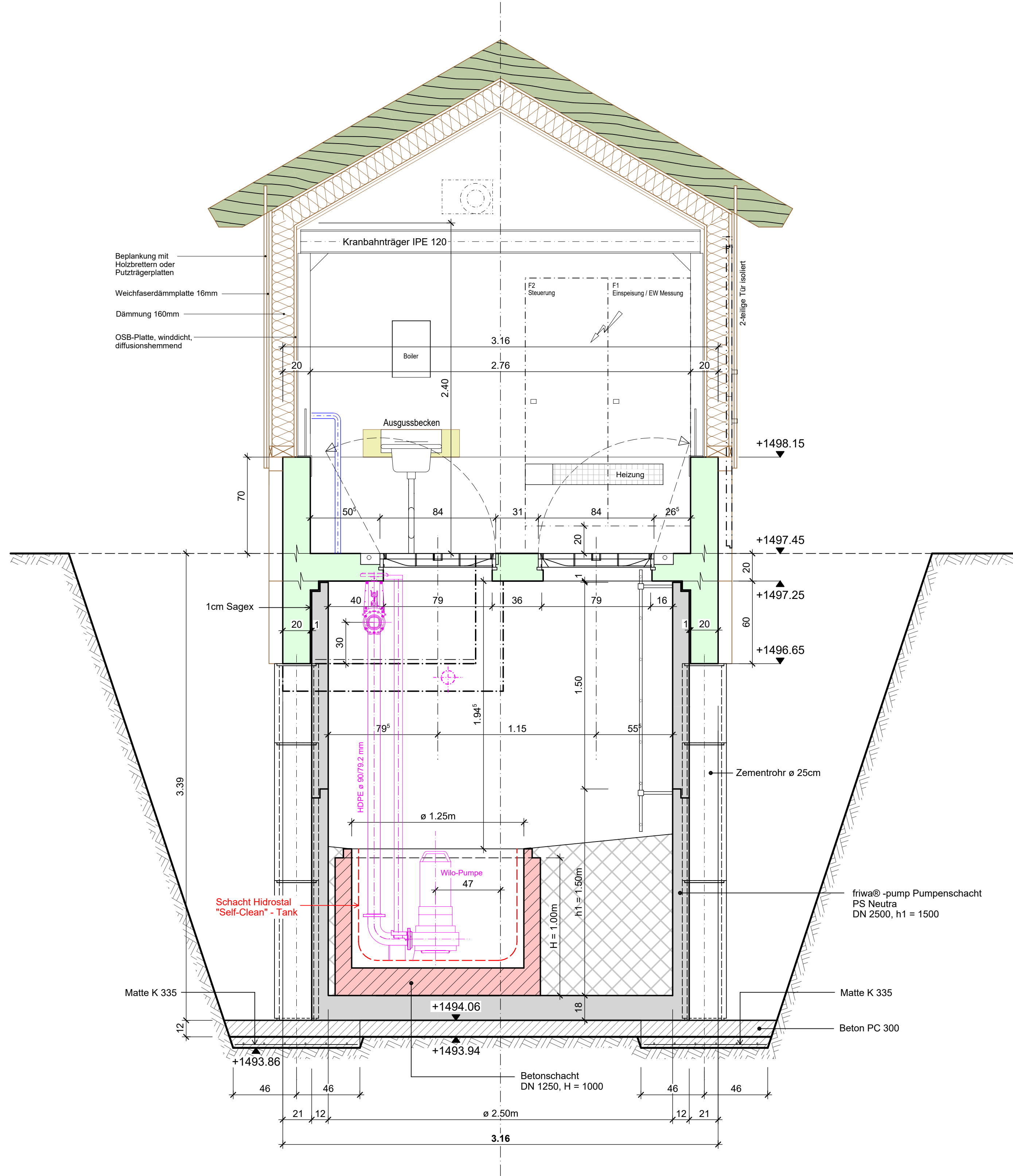
Schnitt A-A 1:20
